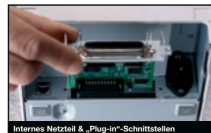
Internes Netzteil & „Plug-in“-Schnittstellen
